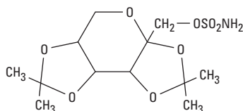
Topiramate
