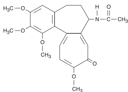
Colchicine
